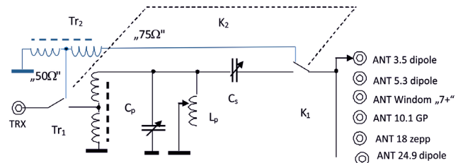
Joonis 1. Antennisobiti põhimõtteskeem
